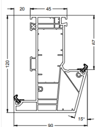
Blendrahmen 120/90 Variant 15° mit Anschlag 19491...
