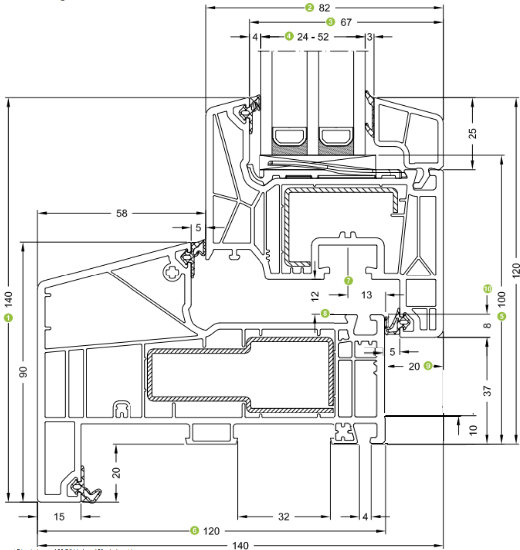
19431... Flügelrahmen 82/83 Vent frame 82/83
