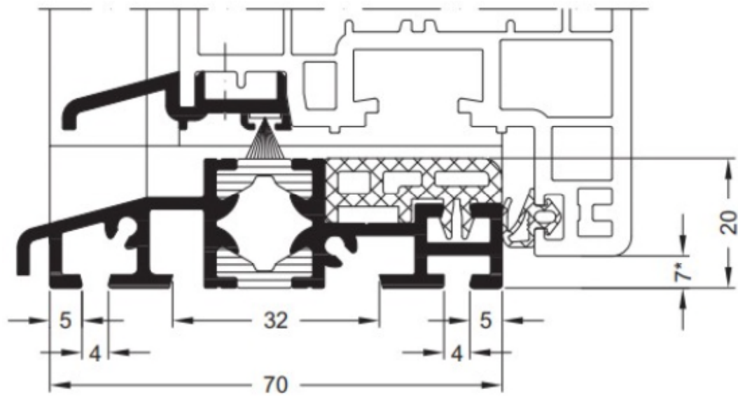
Kombischwelle nach innen öffnend
