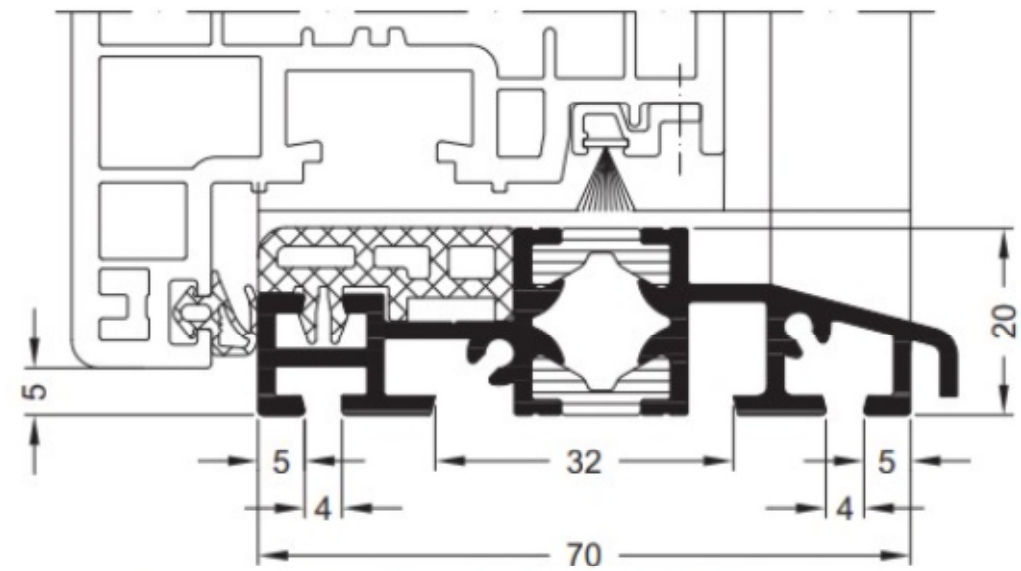
Kombischwelle nach außen öffnend
