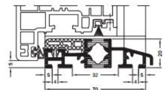
Kombischwelle nach außen öffnend Combination threshold, outward-opening Seuil combiné - ouverture vers l'extérieur Umbral combinado de apertura exterior
